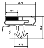
M193 磁2×8
