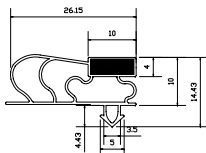
M198 磁3×9
