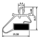
M204 磁3.88×10
