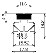
M190 磁3×9
