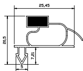
M184 磁4×8
