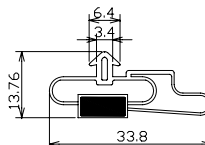
M188 磁3×9
